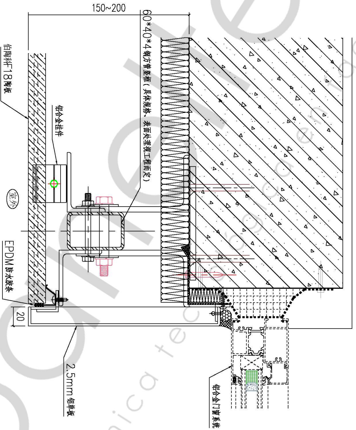
陶板幕墙接铝合金窗侧边节点图
